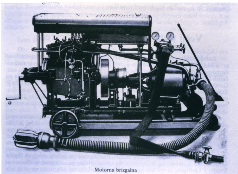
BENZINMOTOR-TURBINENSPRITZE MODELL «MOJSTRANA» ROSENBAUER 1913
