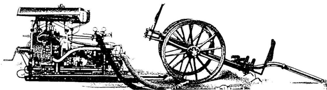
BENZINMOTOR-TURBINENSPRITZE MODELL «MOJSTRANA» ROSENBAUER 1913
